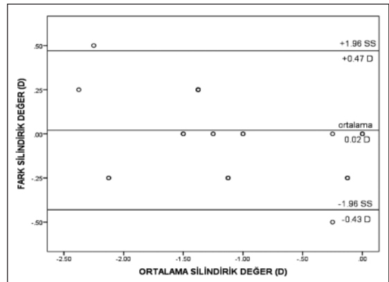
ŞEKİL 3: WASS sikloplejisiz aydınlık ortam ve sikloplejili skiaskopi ile elde edilen silindirik değerlerinin silindirik değerlerinin fark dağılımı \pm 0,49 D arasındadır.
