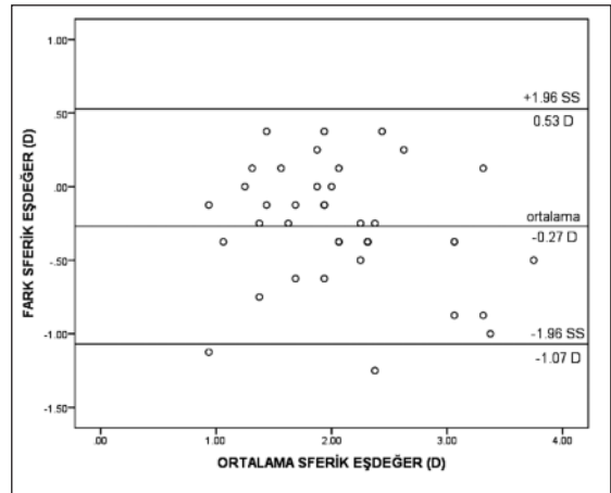
ŞEKİL 2: WASS oto-refraktometre sikloplejili ve sikloplejili skiaskopi ile elde edilen sferik eşdeğerlerinin sferik eşdeğerlerinin fark dağılımı \pm 0,8 D arasındadır.
