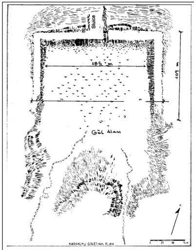
ŞEKİL 2: Karakuyu Barajı'nın planı. (Kaynak: Von Der Osten, H.H., 1933: Fig. 115). 11
