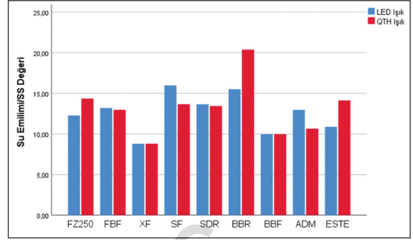
ŞEKİL 2: Su emilimi/Su emilimi değerlerine ait grafik.
