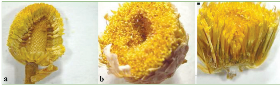
RESİM 1: Papatya numunesinin morfolojisi. a: Matricaria recutita (mays papatyası), b: Aktar papatyası kapitulular
