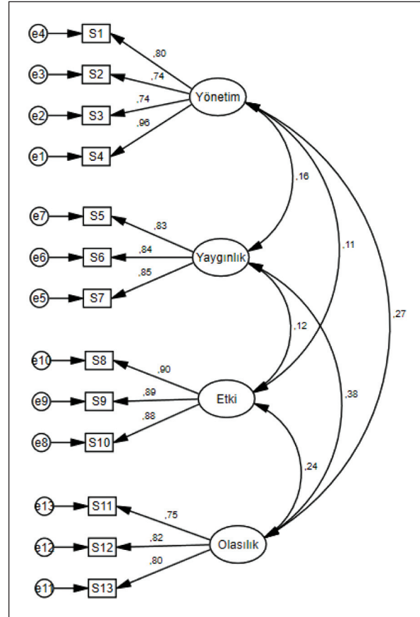
ŞEKİL 2: Sporda Cinsel İstismar Algı Ölçeğine ilişkin doğrulayıcı faktör analizi.
