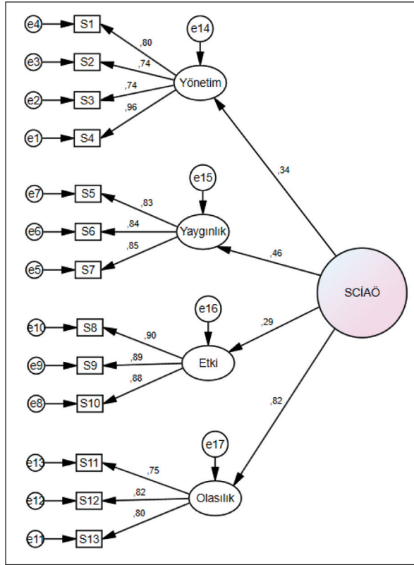
ŞEKİL 3: SCİAÖ'ye ilişkin ikinci düzey (toplam boyut) doğrulayıcı faktör analizi. SCİAÖ: Sporda Cinsel İstismar Algı Ölçeği.
