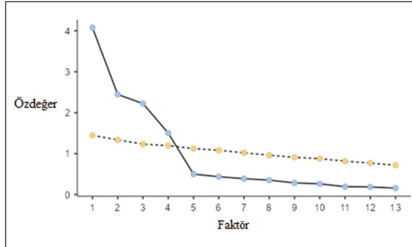
ŞEKİL 1: Faktör çizgi grafiği.
