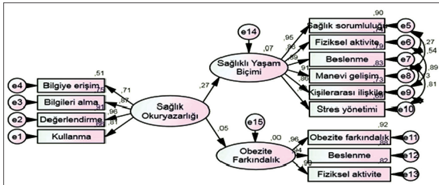
ŞEKİL 1: Sağlık okuryazarlığının sağlıklı yaşam biçimi ve obezite farkındalık üzerindeki etkisine ilişkin yapısal eşitlik modeli.
